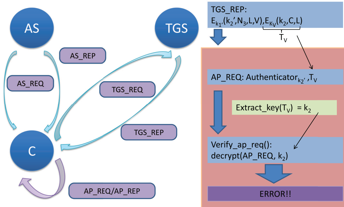
Figure 5: The login process in MIT Kerberos
